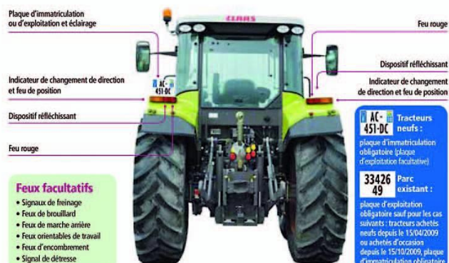
Feux et équipements obligatoires à l'arrière
